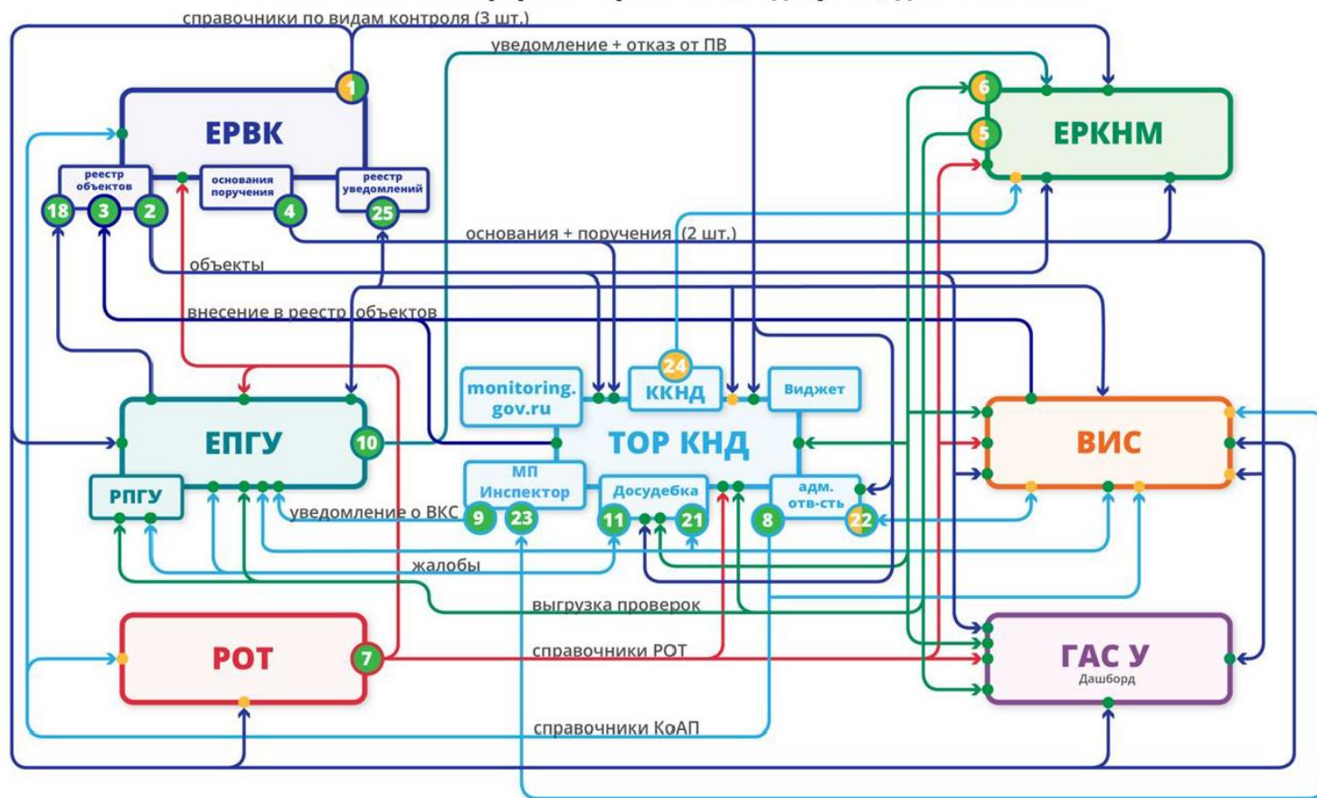
Схема ВС СМЭВ в сфере контрольной (надзорной) деятельности
